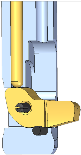
BSF-P: 刀片壳中额外的定位螺栓使刀片的定位更加精确。
