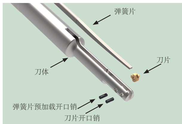
图4: 更换刀片时只需拆除前端开口销即可。
